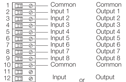
Digital Input/Output Module
